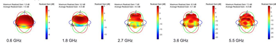
• Antenna a Dipolo installata Verticalmente
