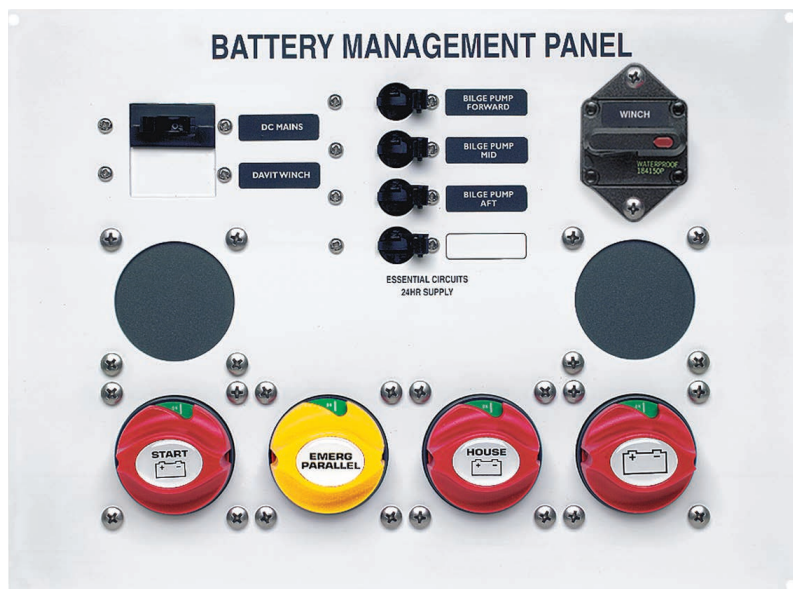
800-MS1
