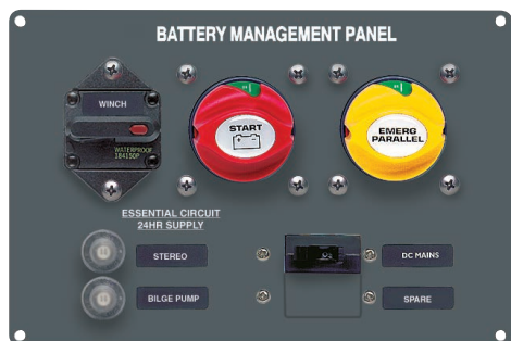
800-MS4
